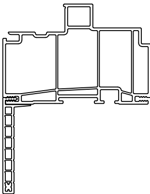
2" FLUSH FIN
